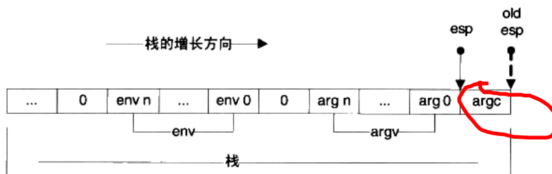
图 11-1 环境变量和参数数组
