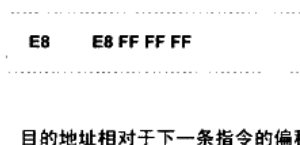
图 7-5 相对偏移调用指令
